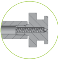
402- HD-Flachkopfnippel HP pan head nipple *405- HD-Flachkopfnippel mit Dichtkonus (vormontiert) HP pan head nipple with sealing cone (pre-assembled)
