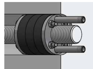
Ringraumpacker, im eingebautem Zustand Annulus packer mounted
